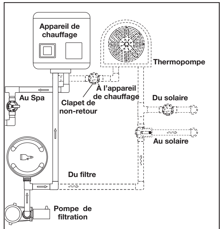
Figure 1. Plomberie pour thermopompe
