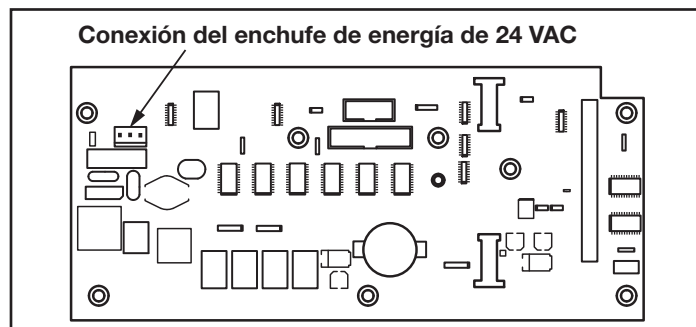
Figura 12. PCB del centro de energía (vista posterior)
