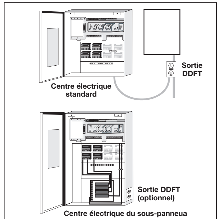
Figure 6. Installation du DDFT pour éclairage sous eau à haute tension
