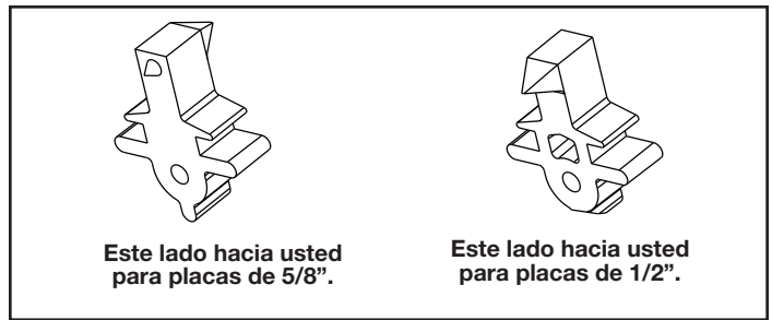
Figura 27. Orientación de los listones
