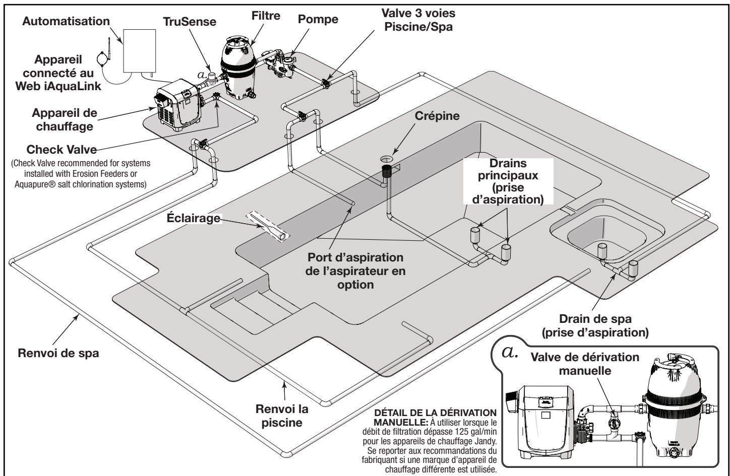
Figure 2. Configuration typique du réseau de canalisation d'eau
