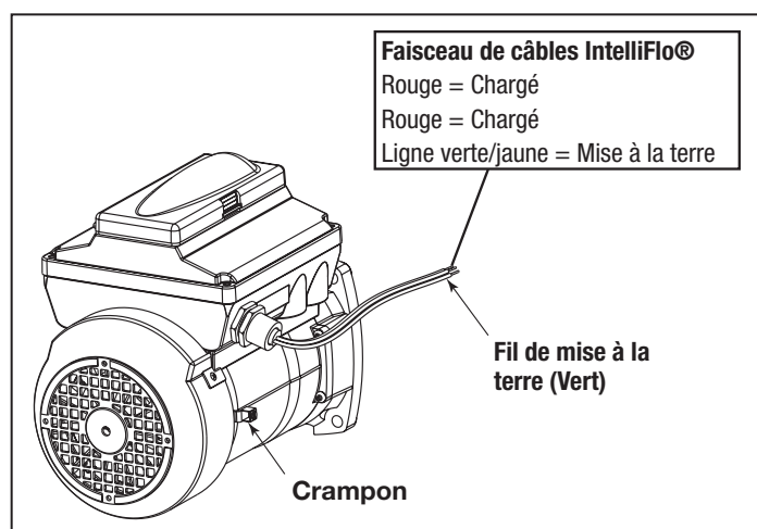
Figure 11. Mise à la masse externe Pentair
